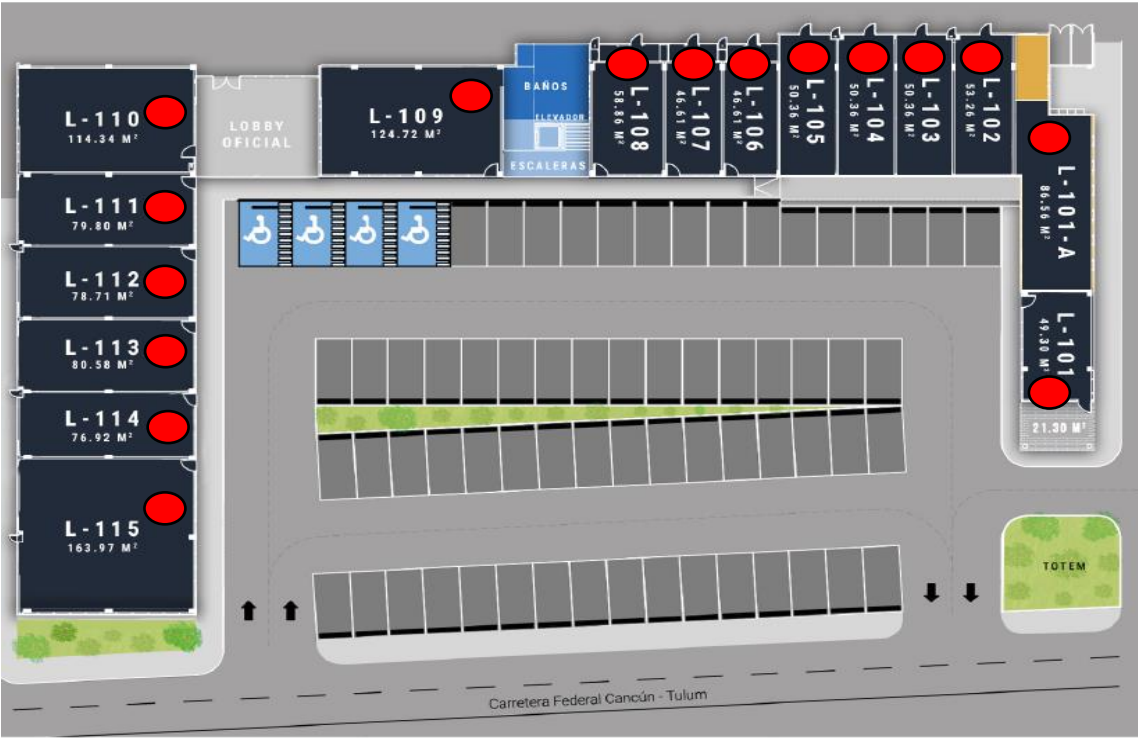
Planta Baja
