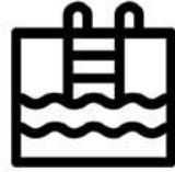
2 ALBERCAS
